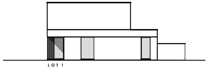
Rechter Zijgevel 1:250
